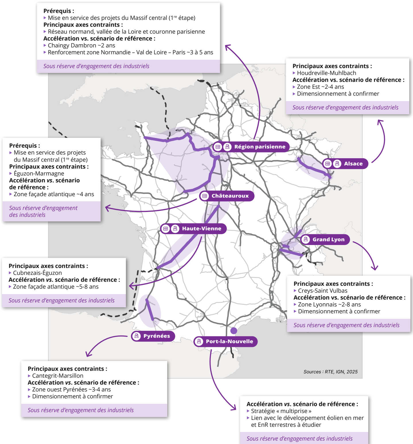
Figure 13 – Options d'accélération de la stratégie réseau THT pour l'accueil de la consommation industrielle d'ici 2030
